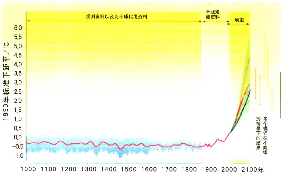
2000~2100年地表温度的变化 (取自IPCC, 2001)
