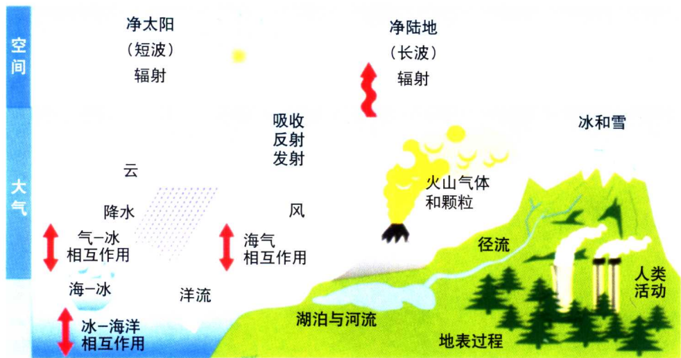
气候系统及其各圈层的相互作用 (取自IPCC, 2001)
