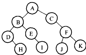
图 1-2 由先序、中序序列确定二叉树的判别过程
