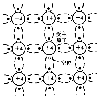
图 1-5 P 型半导体的共价键结构
