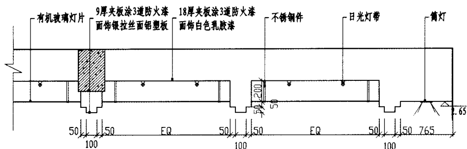
1-1 剖面图
