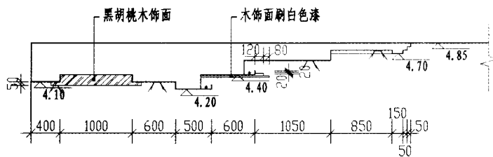
1-1 剖面图
