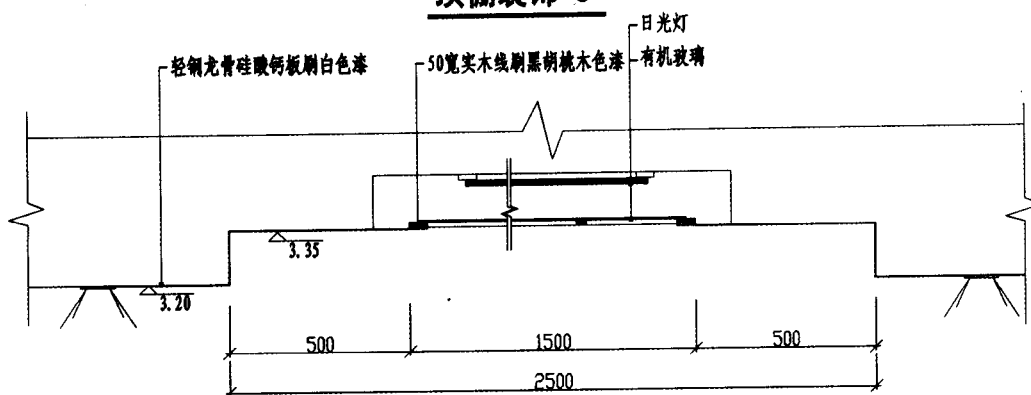
1-1 剖面图
