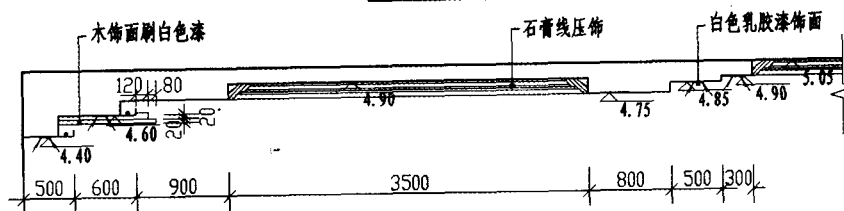
1-1 剖面图
