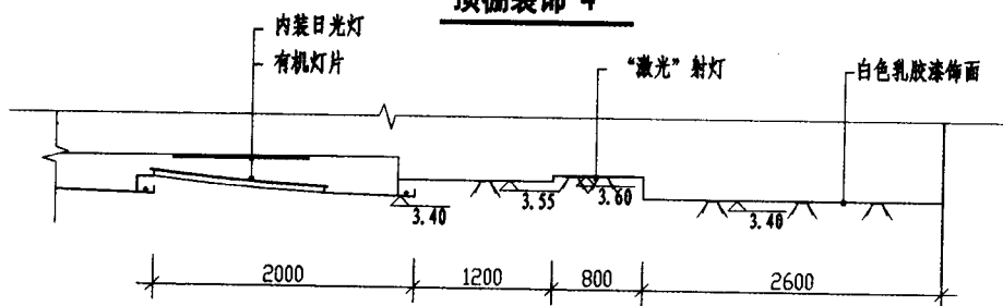
1-1 剖面图
