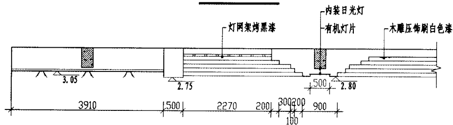
1-1 剖面图
