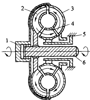
图 1—6 液力变矩器的工作原理
