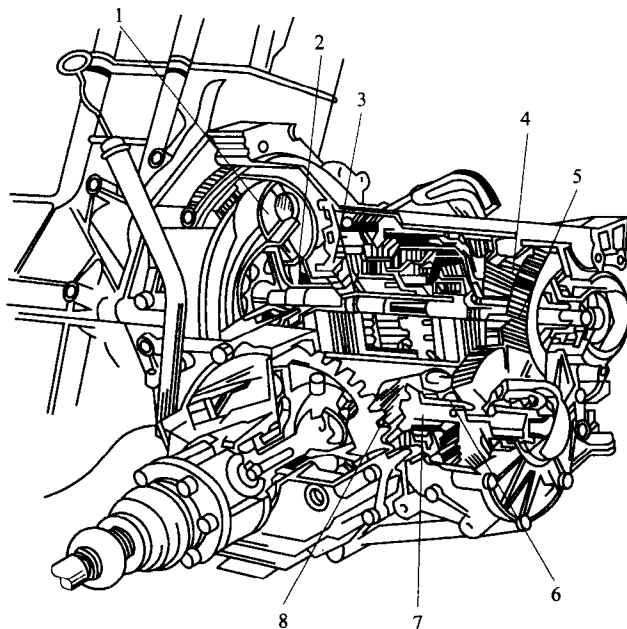
图 1—1 01N 型自动变速器的结构
