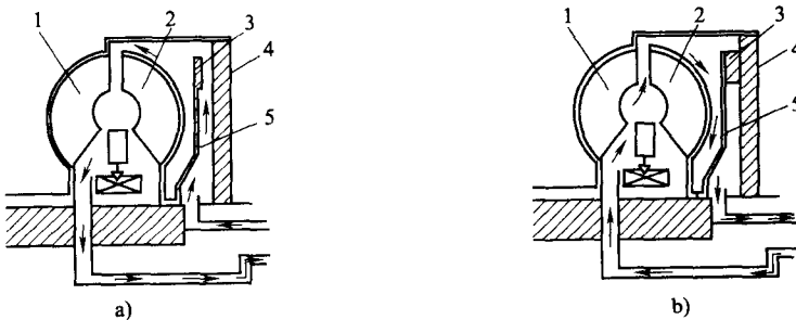
图 1—8 锁止离合器的工作过程
