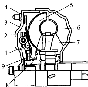
图 1—7 锁止离合器
