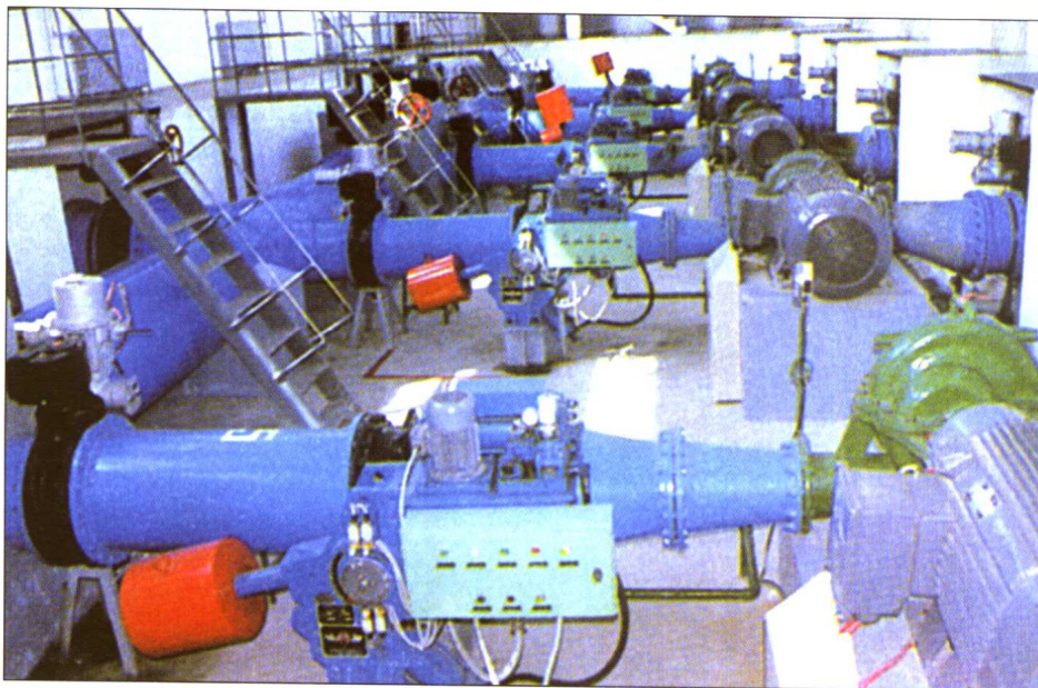
潮白河供水管理所岗山泵站机房
