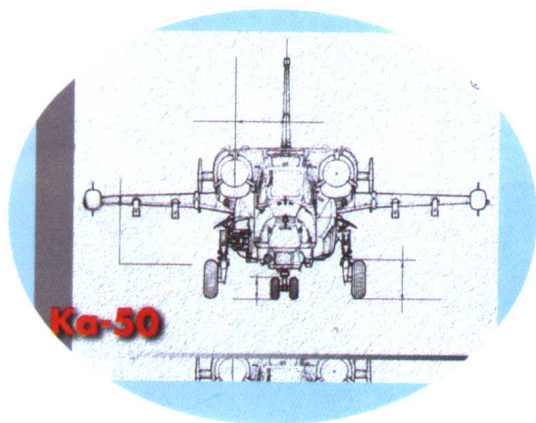
卡-50 结构图
