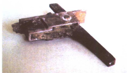
秦王政廿三年造弩机
