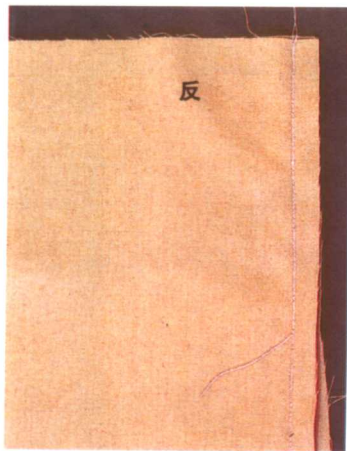
3. 两层衣片正面相对叠合,反面朝外,沿原缝迹线再缉一道。
