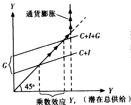
图 0.2(a) 乘数模型
