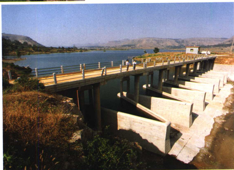
石咀子水库（亚洲中型水库最大的迷宫堰）
