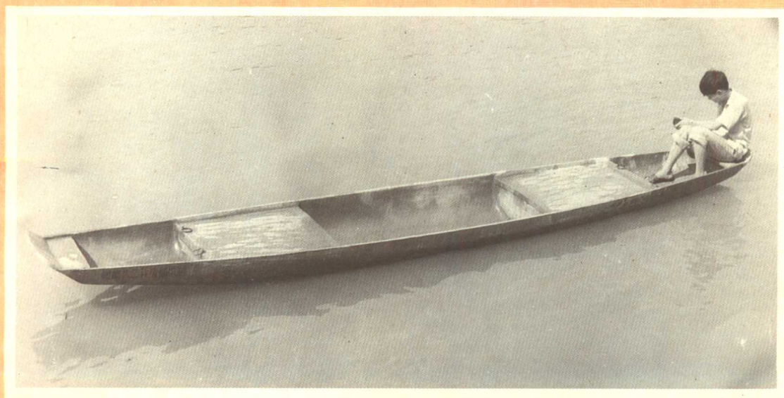
图66 勒流型0.5吨农用水泥艇
