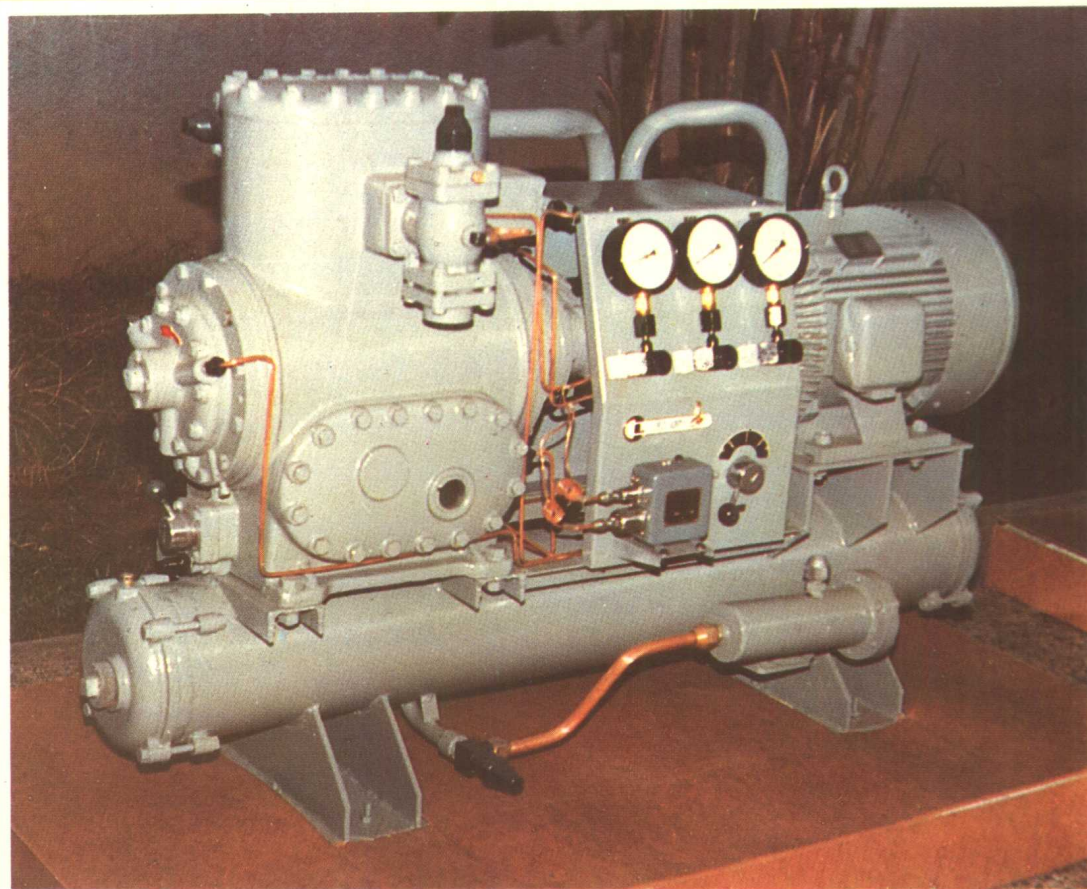
图69 五羊牌2FZ-10氟制冷压缩机
