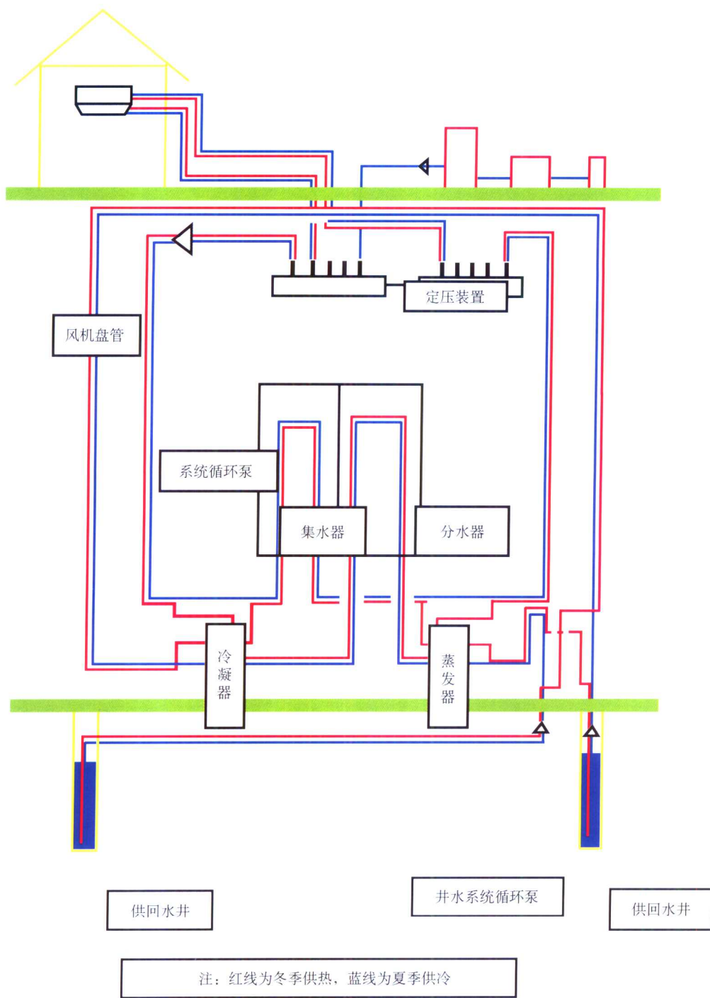
图 14-9-2 水源热泵地温环保中央空调原理图(后勤管理)
