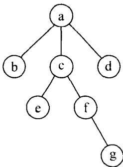
图 1-2 二叉树
