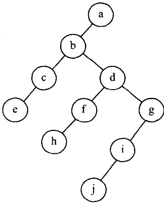
图 1-4 二叉树
