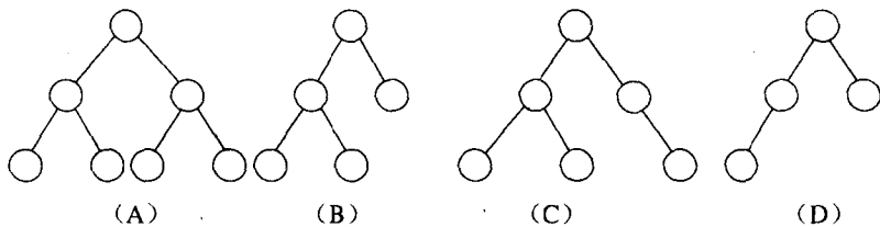
图 1-3 二叉树
