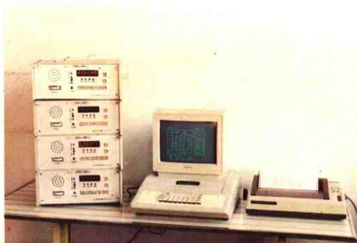
集散型微机配料控制系统
