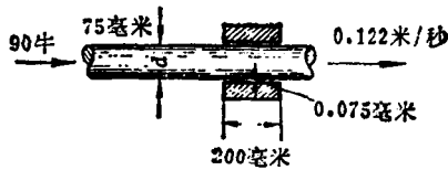
图 1-4 轴与轴套
