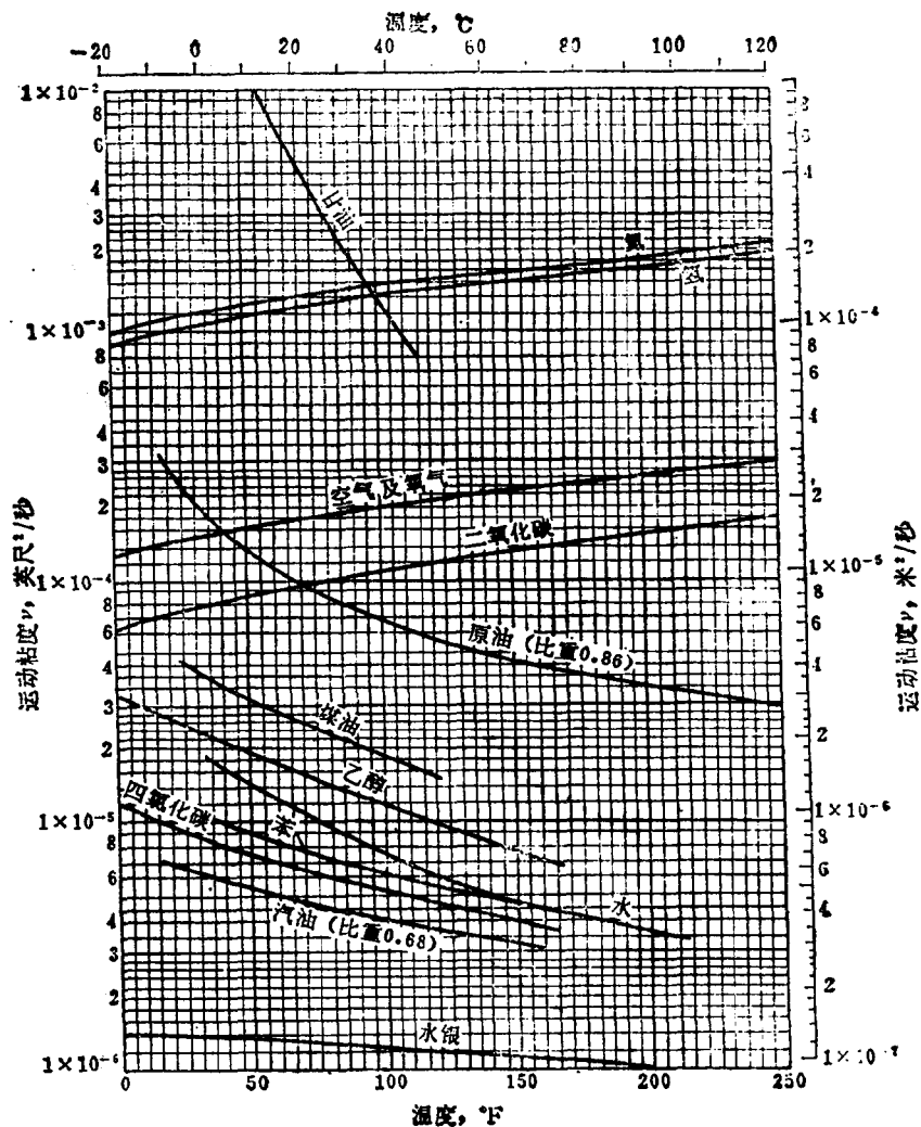
图 1-6 几种液体与气体的运动粘度
