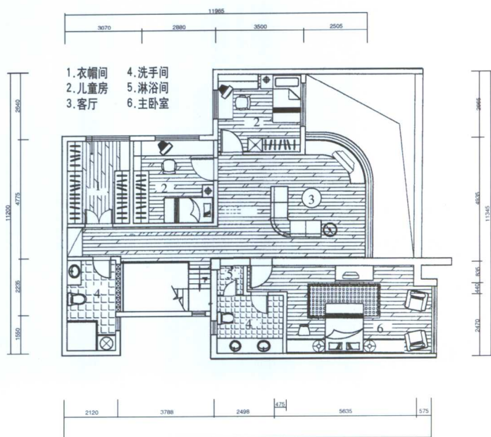
二楼平面图
