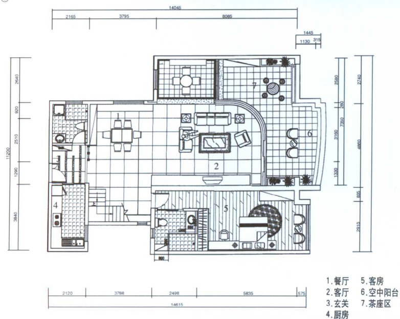
一楼平面图
