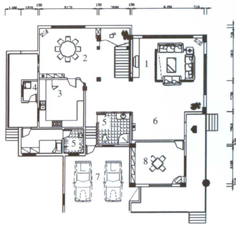
一楼平面图
