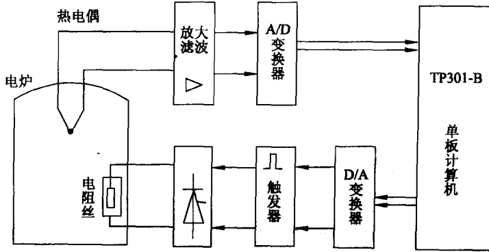
图 1-10 电阻炉温度微机控制系统
