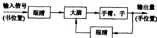
图 1-1 人取书的反馈控制系统方块图
