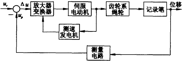
图 1-9 函数记录仪方块图
