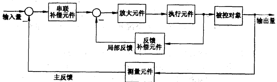
图 1-5 反馈控制系统基本组成
