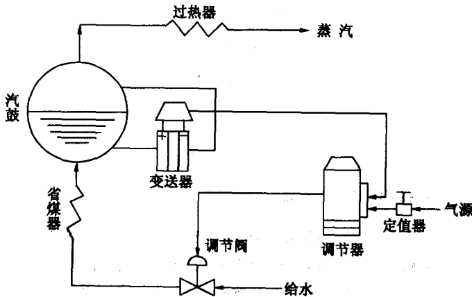
图 1-11 锅炉液位控制系统示意图
