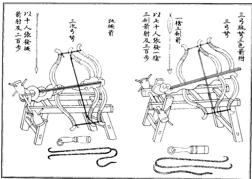
三弓弩圖
