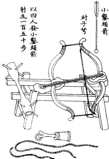
弩圖
