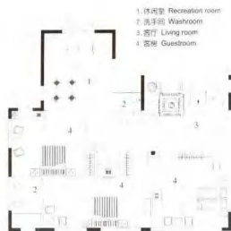
二层平面图 2F plan view
