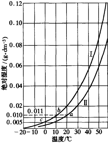
图 1.1 空气湿度与温度的关系曲线 I —— 相对湿度 100% 的饱和曲线 II —— 相对湿度 65% 的饱和曲线
