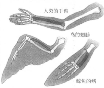
图 1-6a 人、鸟、鲸鱼、人类手臂、鸟的翅膀、鲸鱼前鳍骨骼的比较
