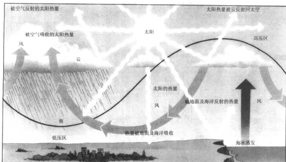
图 1-3 在风云雨雪现象的背后,是水的三相变化的循环规律
