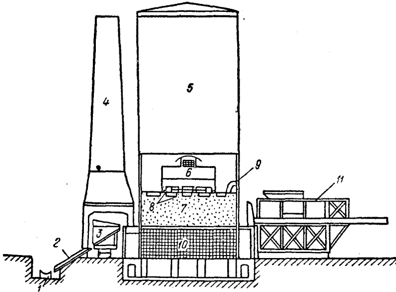
圖 1 煉焦爐斷面圖
