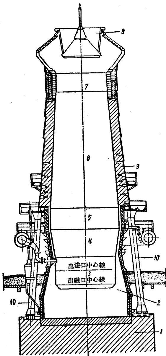
圖 2. 高爐斷面圖 1—基礎；2—爐底；3—爐缸；4—爐腹；5—爐腰；6—爐身；7—爐頂；8—進料裝置； 9—爐殼；10—柱（爐身支柱）
