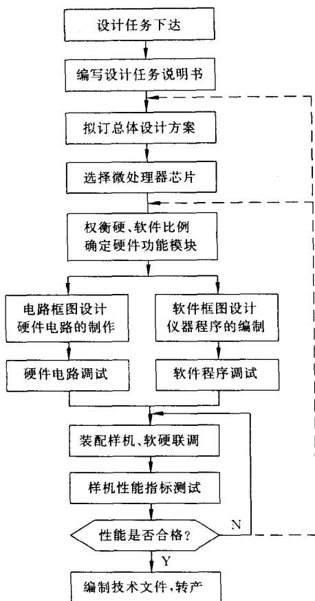
图 1-5 设计、研制智能仪器的一般过程
