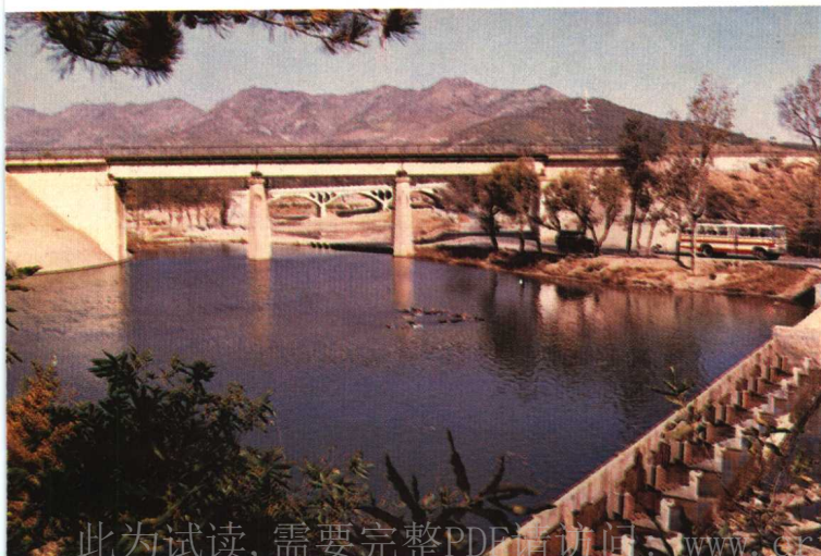
平度县泽河上的自动翻板栏河闸
