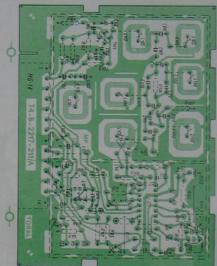
M P 1001 图象中放印刷电路板图
