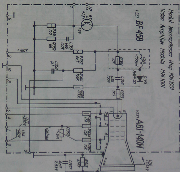
MW1001 视放电路图
