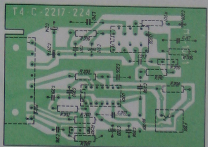
M F 1001 伴音印刷电路板图
