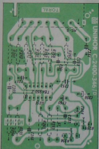
M S 1001 同步及行扫描印刷电路板图
