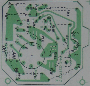
MW1001视放印刷电路板图
