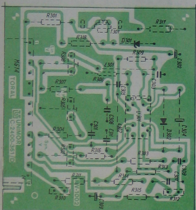
M V 1002 帧扫描印刷电路板图
