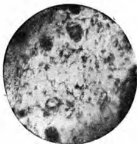
图9,a 混合料含碳量3.5%时的磁铁矿颗粒 反光 (放大225倍)
