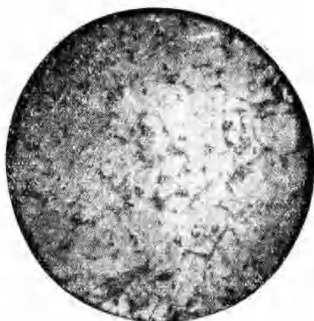
图9,c 混合料含碳量4.5%时的磁铁矿颗粒 反光(放大225倍)
