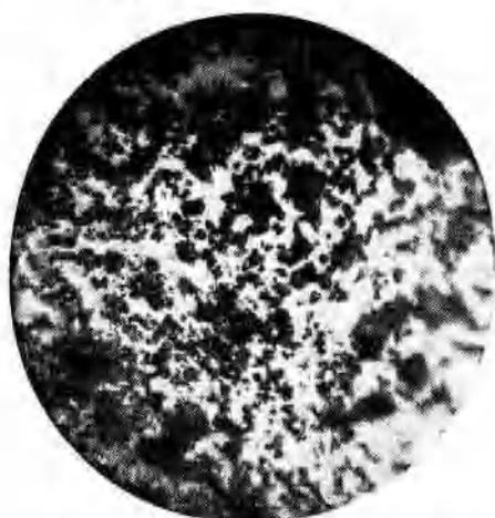
图4,e 碱度2.54,磁铁矿和铁酸钙不规则连晶反光(放大225倍)
