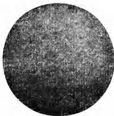
图9,d 混合料含碳量5.0%时结晶粗大的磁铁矿颗粒 反光(放大225倍)
