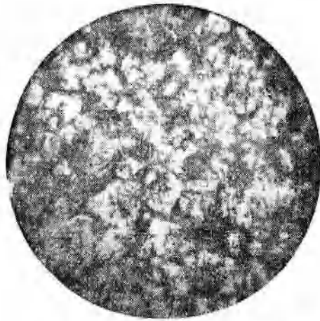
图6. b 混合料含碳3.5% 粘结物为玻璃质反光(放大225倍)
