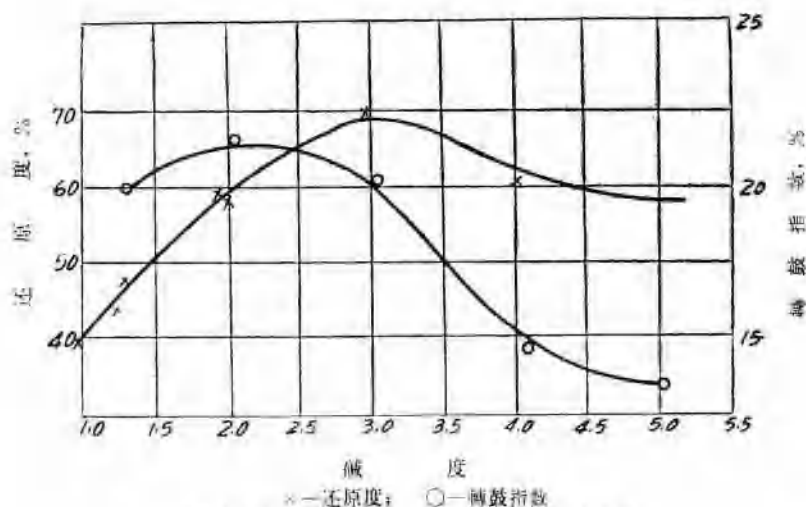
图10 不同碱度的凹山烧结矿的强度及还原性
