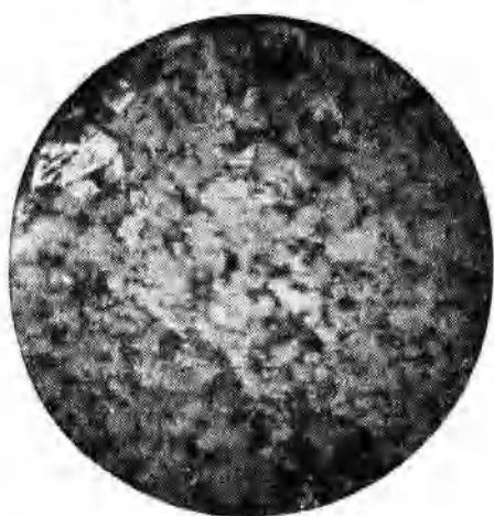
图4,c 碱度1.85,铁酸钙的板状晶体反光(放大225倍)
