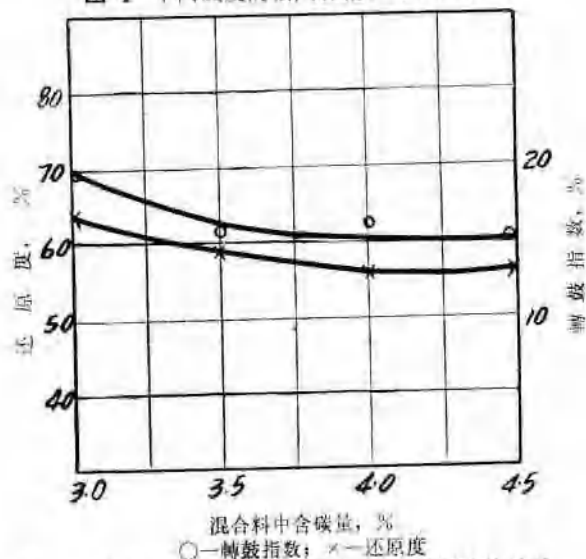
图5 混合料中含碳量与烧结矿强度、还原性的关系
