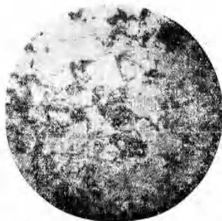
图7.b 碱度1.41, 次生磁铁矿的镶边结构 反光(放大225倍)
