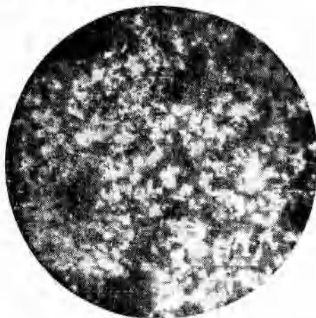
图6. a 混合料含碳3.0%, 磁铁矿结晶不规则, 粘结物是玻璃质反光(放大225倍)
