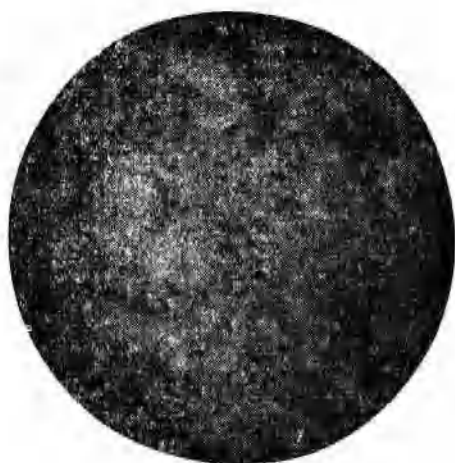
图7.a 碱度1.41磁铁矿的集合体反光 (放大225倍)
