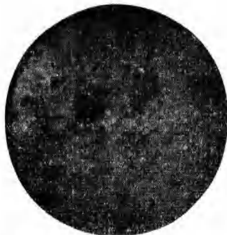
图7.c 碱度5.0, 磁铁矿和铁酸钙的不规则连晶反光(放大225倍)
