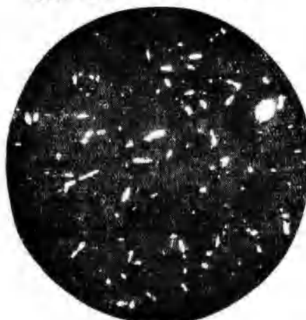
图4,f 碱度2.54,正硅酸钙的短柱晶体透射光(放大90倍)
