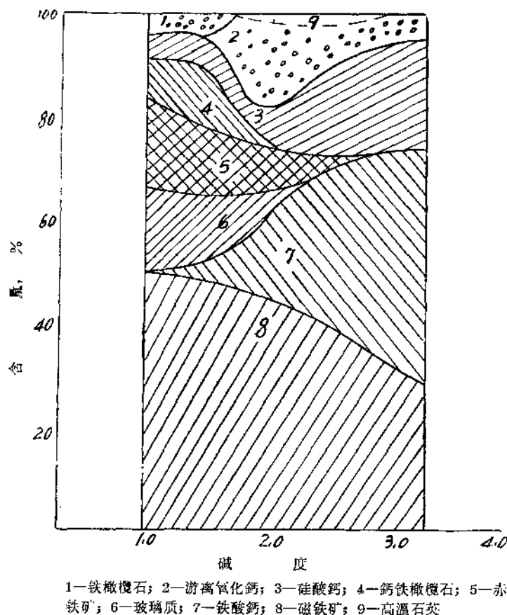
图 2, a 不同碱度鞍山烧结矿的矿物组成
