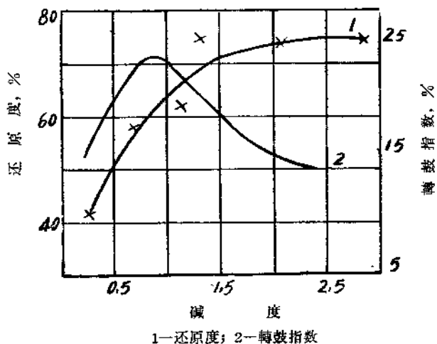
图 3 鞍山烧结矿碱度和还原性的关系
