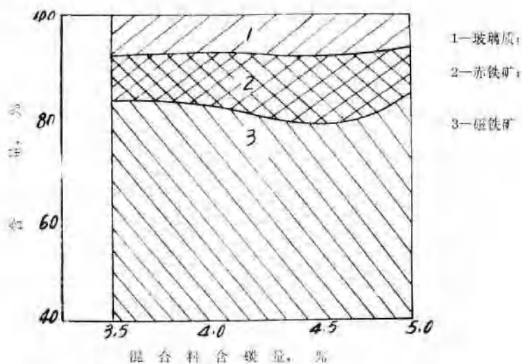
图8,b 混合料含碳不同时团山烧结矿的矿物组成
