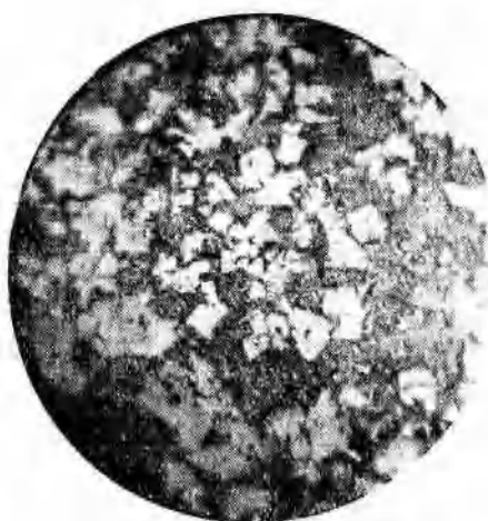
图6,c 混合料中含碳4.0 磁铁矿结晶比较好,粘 结物为玻璃质及钙铁橄榄石反光(放大225倍)
