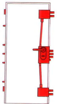
门锁结构
