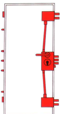
门锁结构
