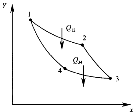
图 1-1 任意力学变量的卡诺热机
