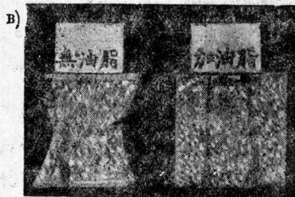
第 3 圖 混凝土立方試驗時計算的 (a) 與實際的 (b) 載荷情形及破壞情形 (b)
