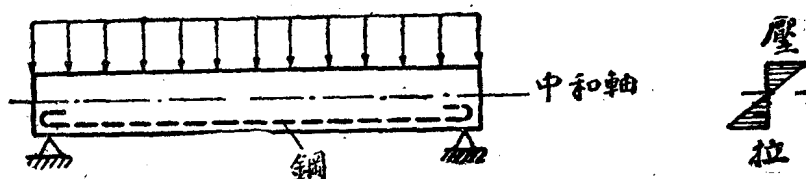
第1圖 受彎構件的工作草圖
