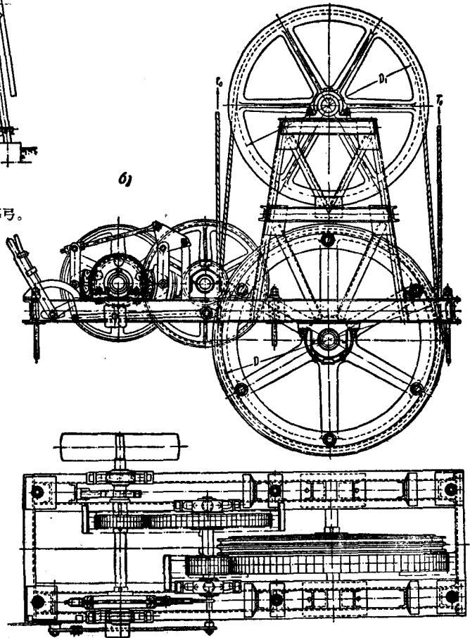
圖4 帶凹槽磨擦輪的牽引索傳動裝置: а—水平的; б—垂直的。
