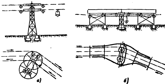
圖23 單索架空道線路轉角站： a) 半自動的；b) 用剛性站線的非自動的。
