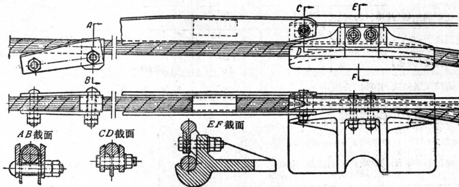
圖14 承載索用的偏向導靴。
