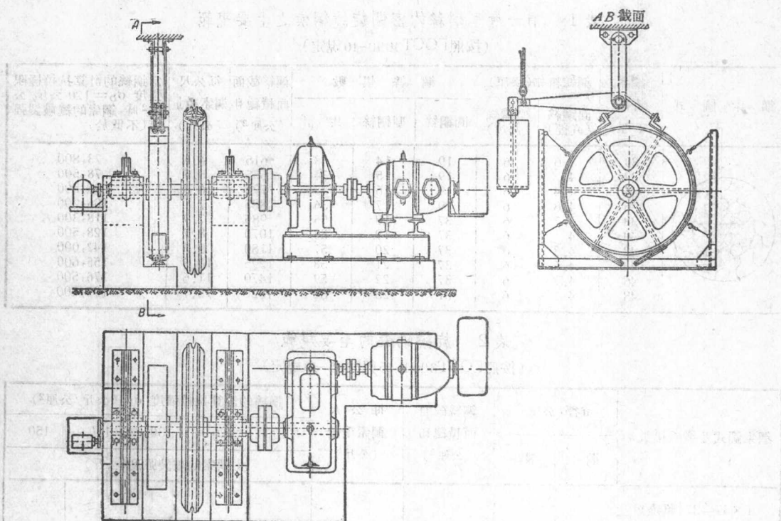
圖 5 帶有索夾的垂直滑輪牽引索傳動裝置。
