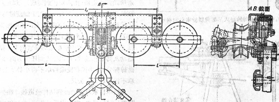
圖 8 有重力索夾的四輪跑車。
