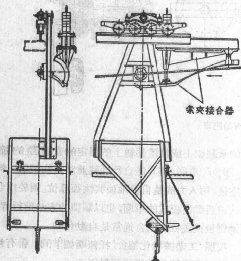
圖11 有摺合的車廂側板與橫桿索夾的料車。
