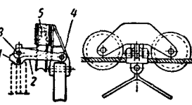
圖22 用鉗口索夾的單索架空道料車的跑車。
