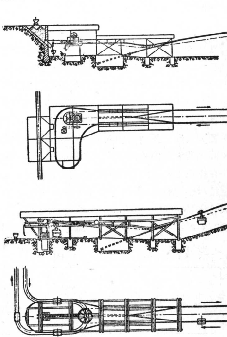
圖12 雙索架空道裝貨終點站。
