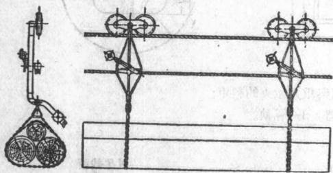
圖10 有輸送圓木用的鏈式吊架與螺旋索夾的料車。
