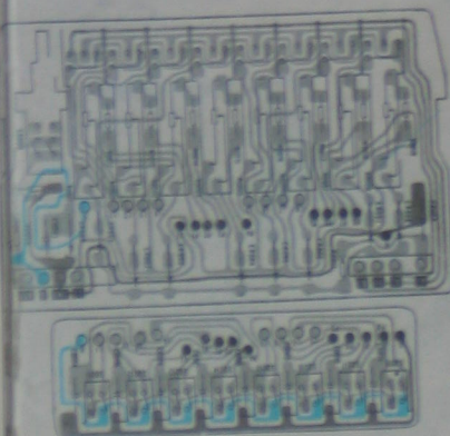
选台单元印刷电路板
