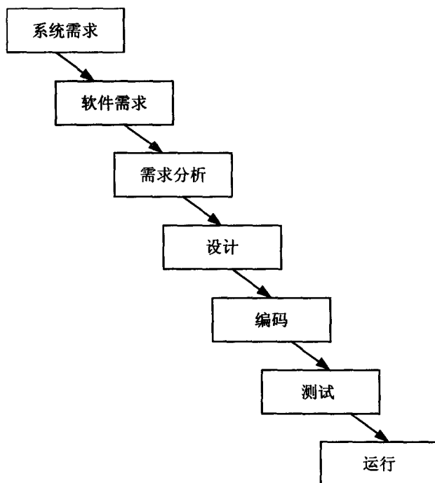
图 1.3 瀑布模型
