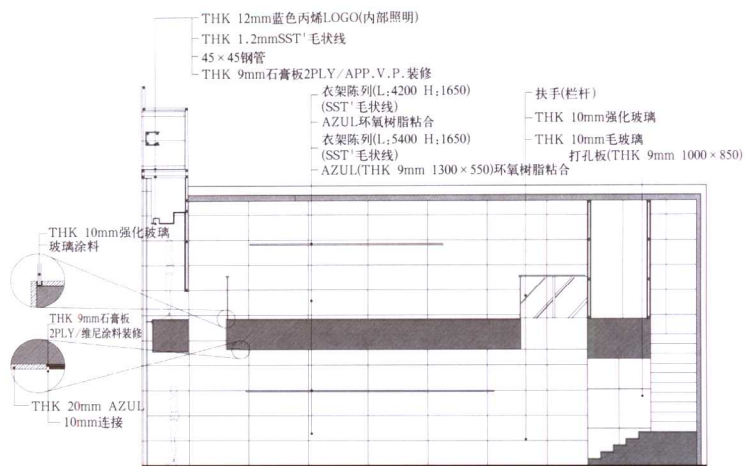
截面图
