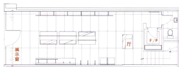
平面图
