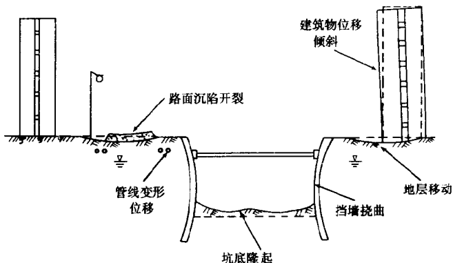
图1 基坑开挖对周围环境的影响
