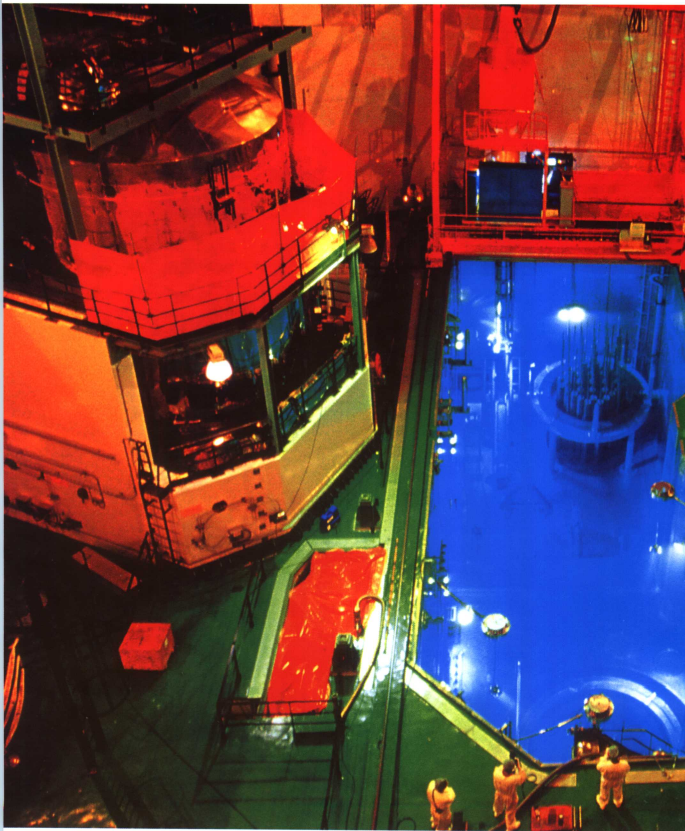
在反应堆厂房内进行装料操作
