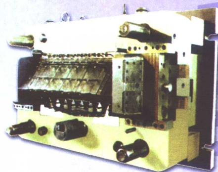
整体梯级压铸模
