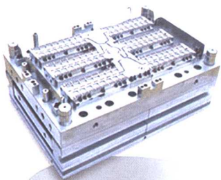
塑封封装模具(单缸)
