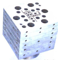
挤出模头
