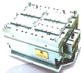
塑封封装模具(多缸)
