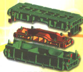
三维模具设计
