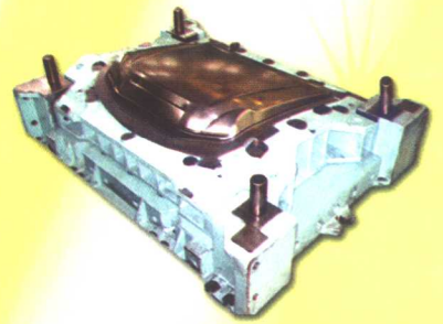
发动机罩外板拉伸模
