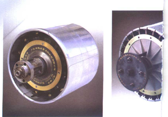
→ 辐射扩张及机械折叠成型鼓
