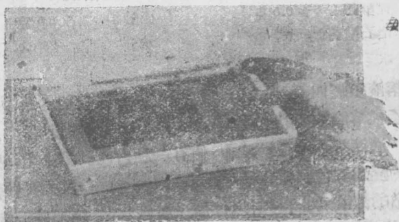
圖 4. 銀沉積於放在溶液中的玻璃片上。
