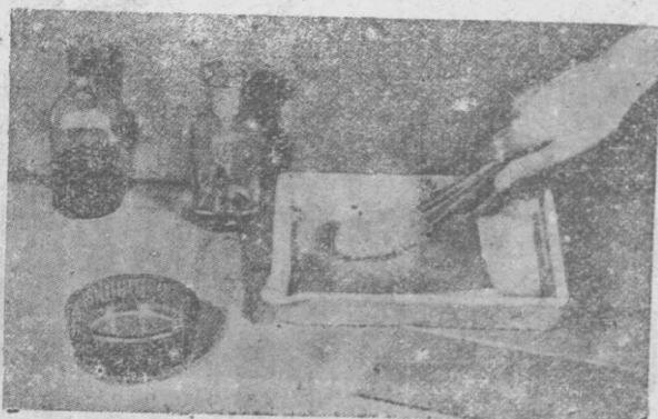
圖3. 玻璃在塗銀之前，需用化學溶液洗淨。圖示兩根玻璃棒夾着一塊棉花，用硝酸把玻璃措拭。
