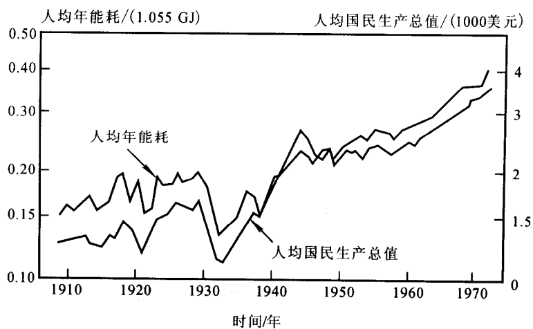
图 1-1 1909—1973 年美国国民生产总值和能源消耗关系曲线
