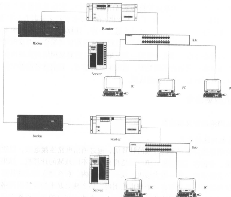
图 1-1 计算机网络示意图
