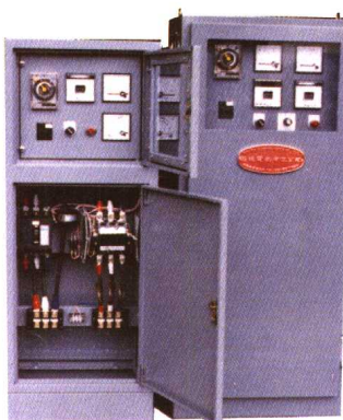
電磁式開關 溫度控制盤
