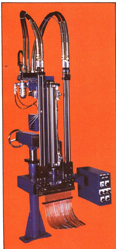
離型劑自動噴霧裝置
