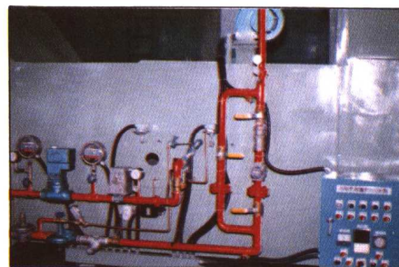
瓦斯燃燒室
