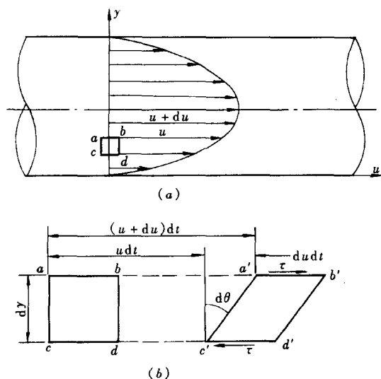
图 1-1 流体质点的直角变形速度
