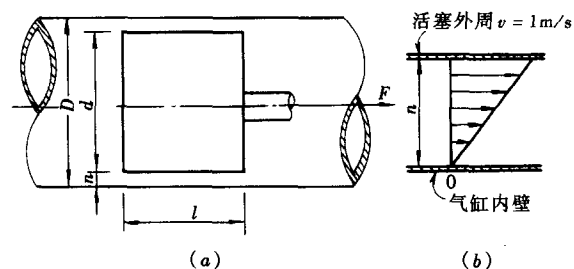
图 1-2 活塞运动的黏性阻力
