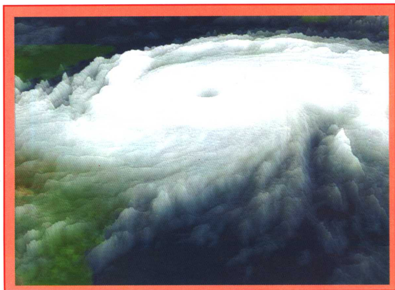
台风眼和台风云
