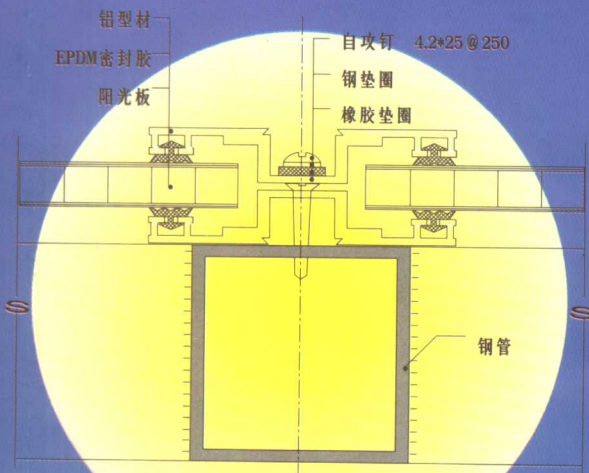
标准连接节点
