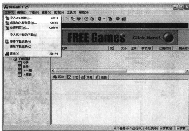
图1-2 “文件”菜单
