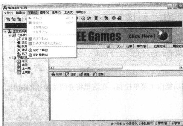
图1-3 “下载”菜单
