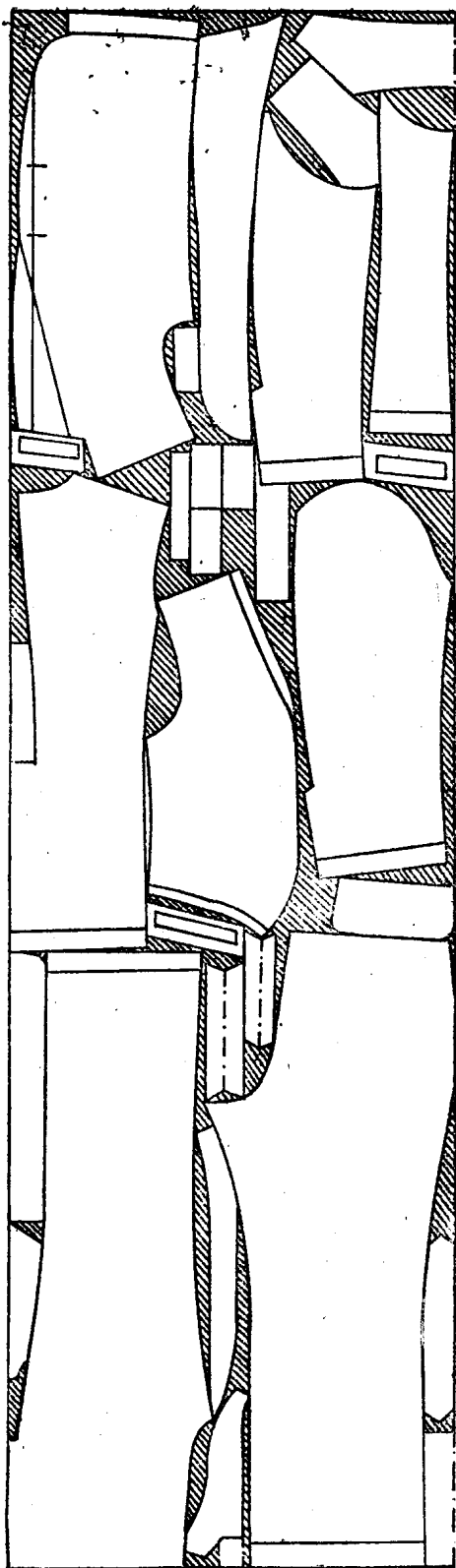
165/88 男单排扣(三件套)西装排料示意图
