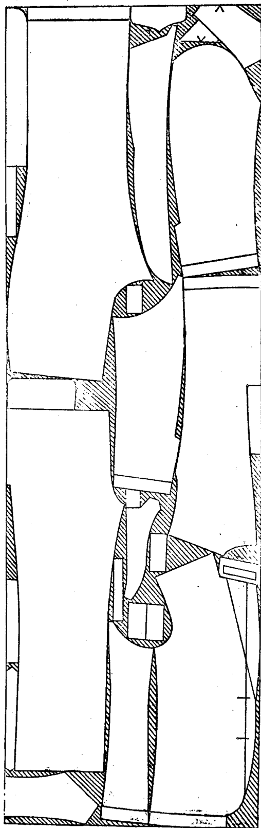
165/88 男单排钮(二件套)西装排料示意图
