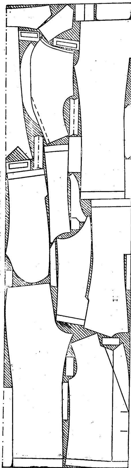
165/88 男双排钮(三件套)西装排料示意图
