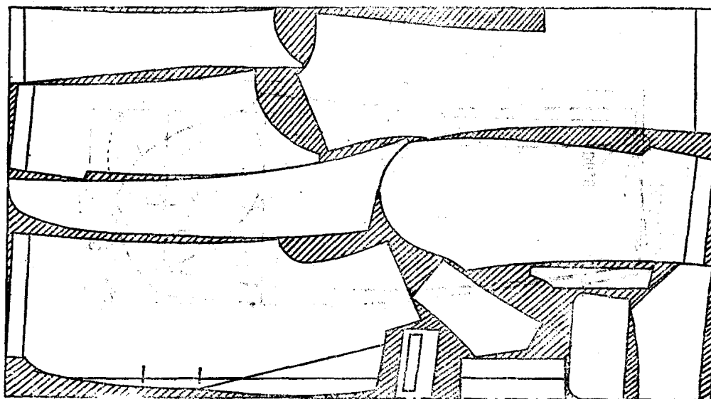
160/85 男单排钮西上衣排料示意图
