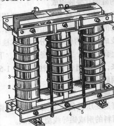
图 1-5 三相三柱式变压器铁芯
