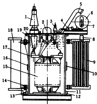
图 1-2 变压器结构
