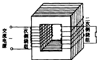
图 1-1 变压器基本原理图
