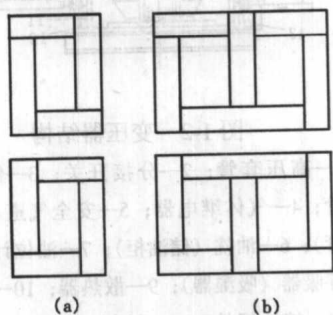
图 1-4 变压器铁芯的交叠装配 (a) 单相变压器; (b) 三相变压器
