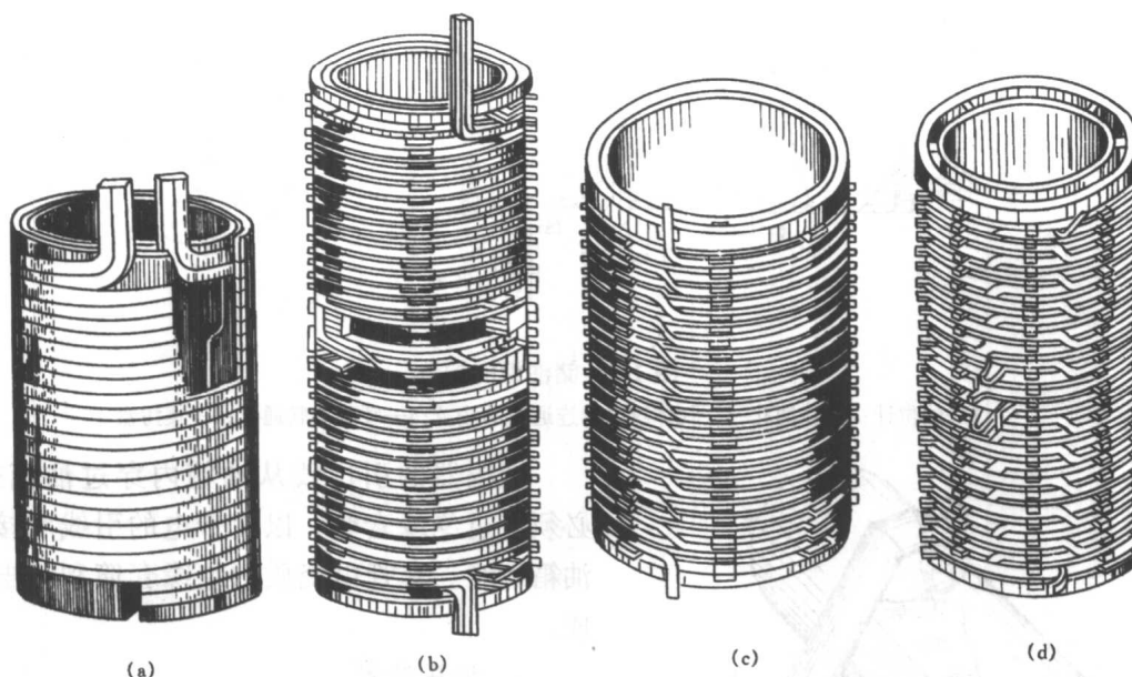
图 1-6 变压器绕组形式
