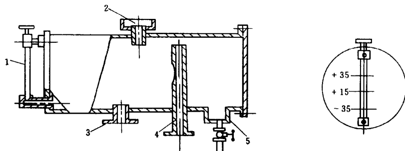
图 1-7 储油柜的构造
