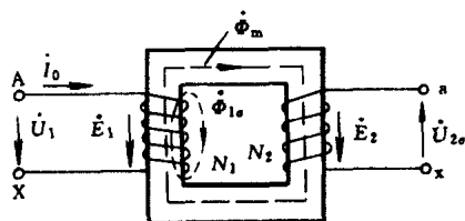
图 1-9 单相变压器空载运行时的示意图
