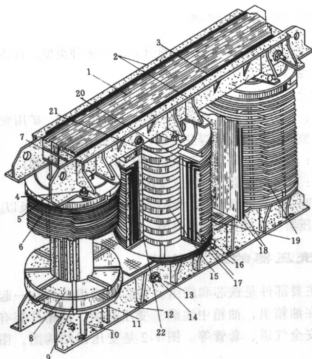
图 1-3 变压器器身结构
