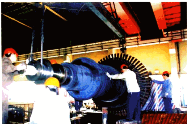
◀ 汽轮机大修
