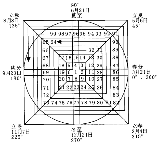
图 1-2 江恩数字正方形与圆周
