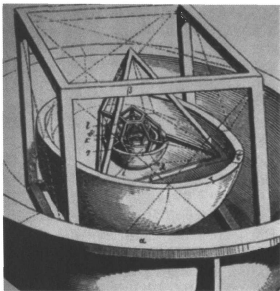
图 1-1 开普勒的宇宙模型
