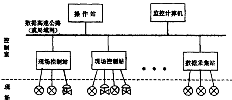
图 1-4 传统 DCS 的基本结构
