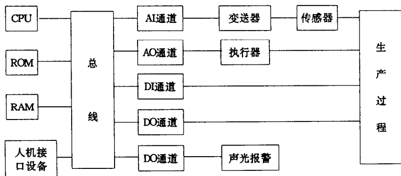
图 1-3 基本的计算机控制系统
