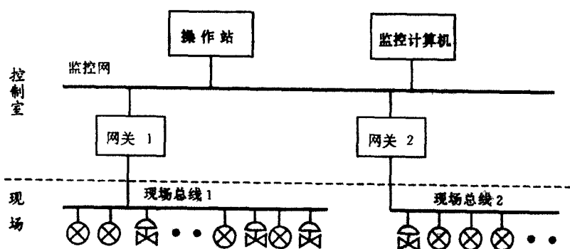
图 1-5 FCS 典型结构
