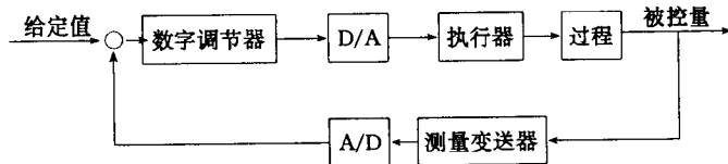
图 1 2 计算机单回路控制系统的结构
